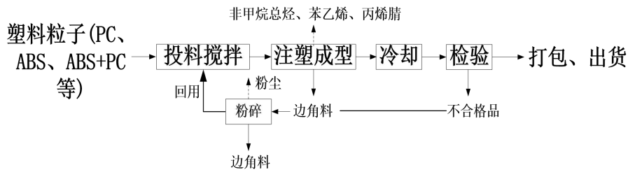
图 2-2 模组工艺流程及产污环节图
