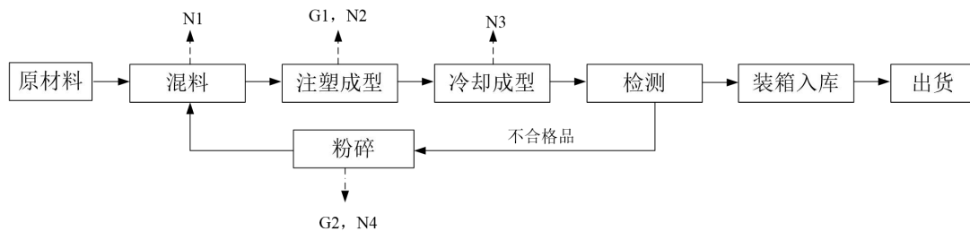
图 5-1 塑制品件生产工艺流程图
