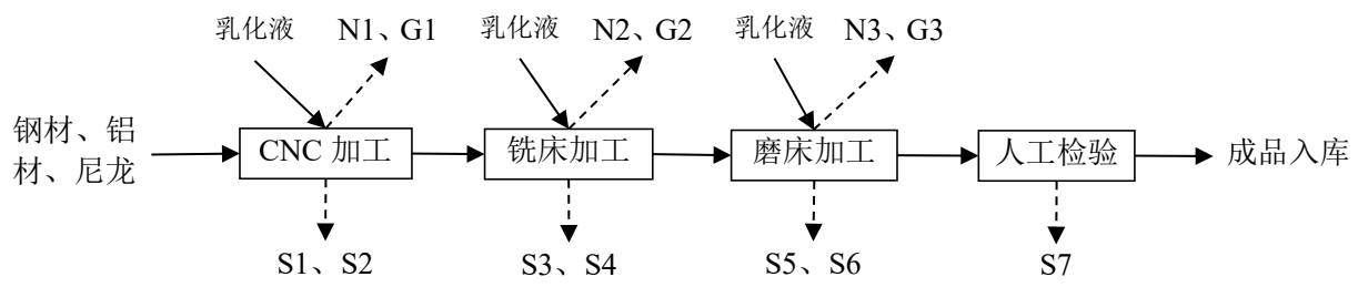
图 5-1 生产工艺流程及产污环节图
