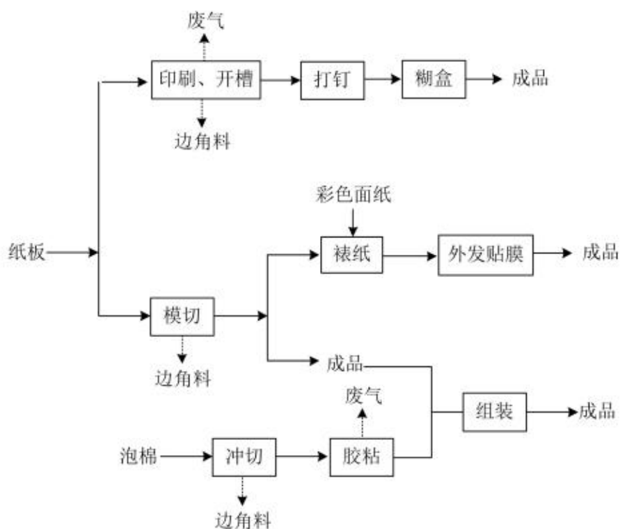
图 2-3 纸质包装制品生产工艺流程
