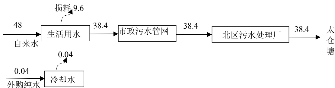
图 5-2 水平衡图 t/a
