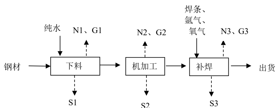
图 5-1 生产工艺流程及产污环节
