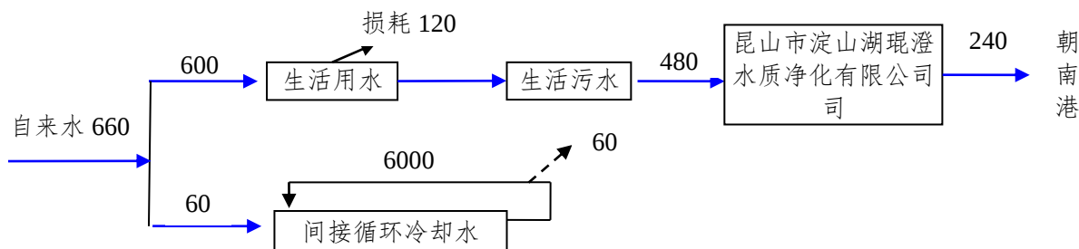
图 2.1-1 水平衡图 单位 t/a
