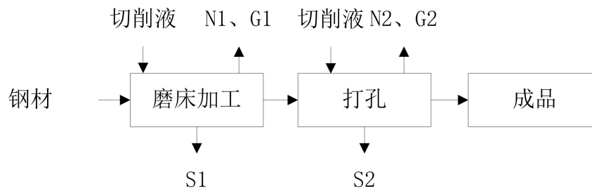
图 5-1 生产工艺流程及产污环节
