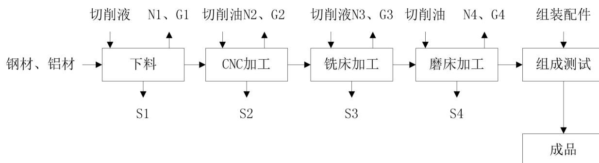
图 5-1 生产工艺流程及产污环节
