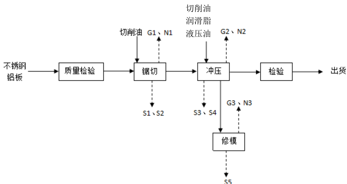
图 5-1 五金冲压件生产工艺流程及产污环节图
