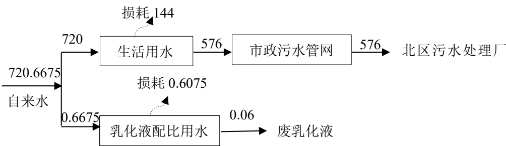
图 5-3 本项目水平衡图（单位：t/a）
