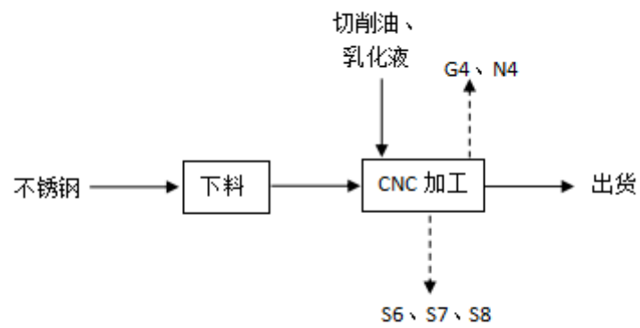
图 5-2 模具（用于冲床）生产工艺流程及产污环节图
