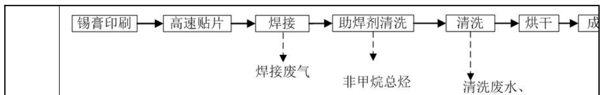
图 2-10 电路板生产工艺流程及产污环节图
