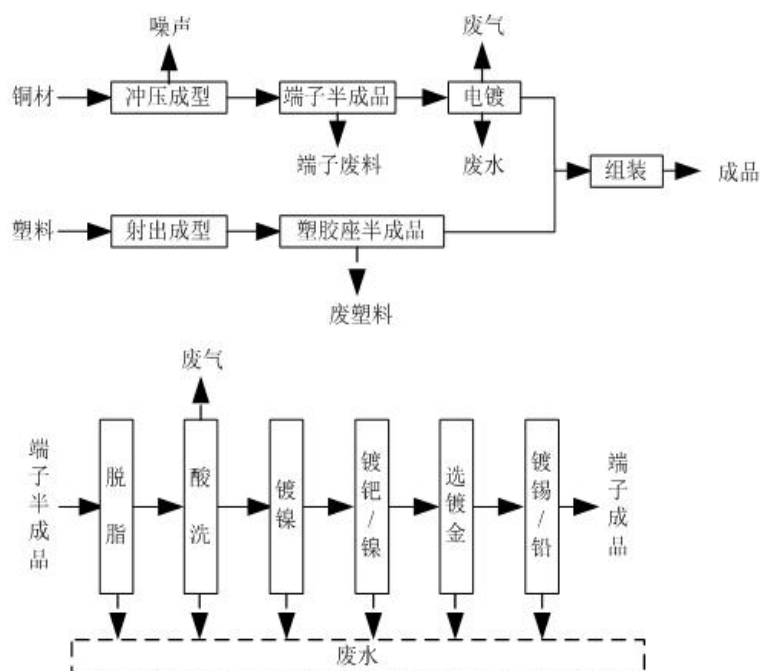
图 2-3 连接器生产工艺流程及产污环节图
