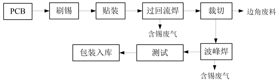
图 2-6 印刷电路板工艺流程及产污环节图
