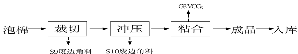
图2-8 现有项目生产工艺流程及产污环节图
