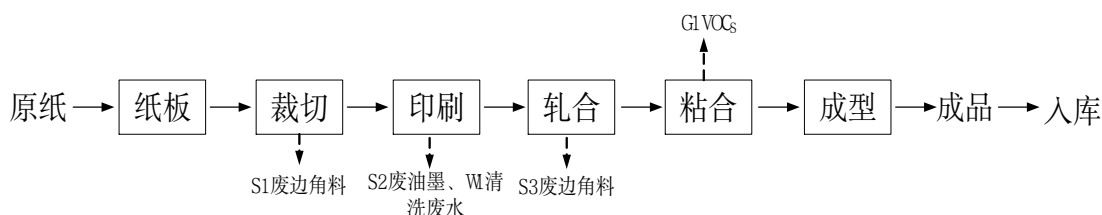
图 2-5 现有项目生产工艺流程及产污环节图
