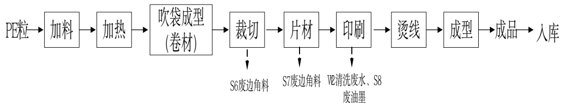
图2-7 现有项目生产工艺流程及产污环节图
