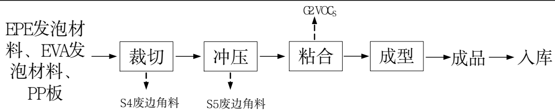
图 2-6 现有项目生产工艺流程及产污环节图
