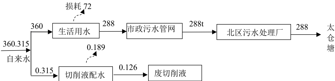
图 5-2 水平衡图 t/a
