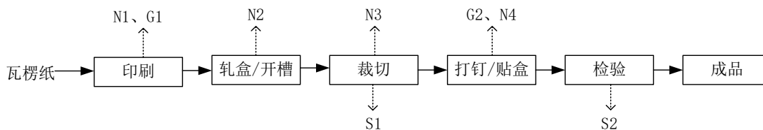
图 2-2 包装纸箱生产工艺流程图
