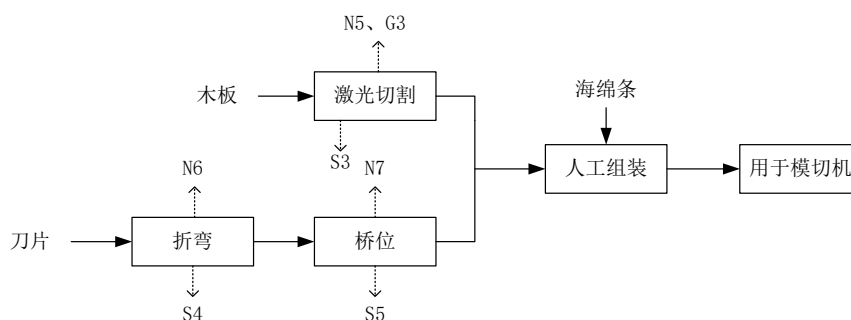
图 2-3 刀模生产工艺流程图
