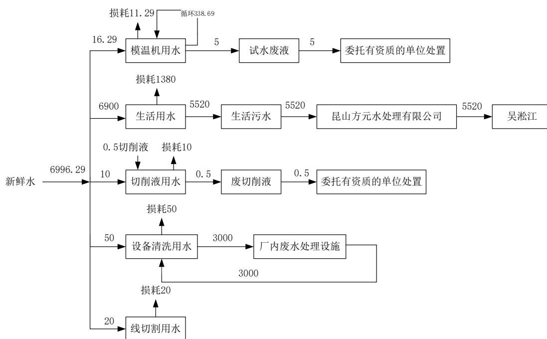
图 2-1 全厂水平衡图
