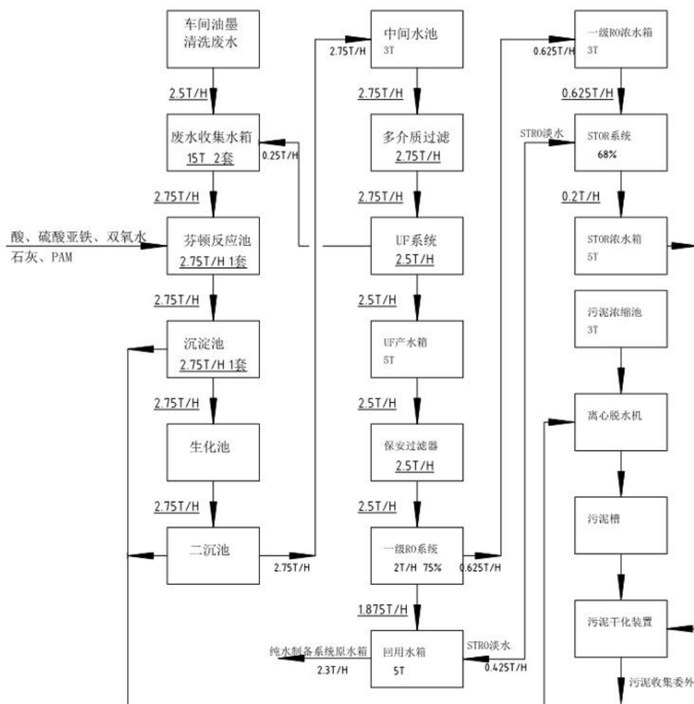
图 4-1 废水处理工艺
