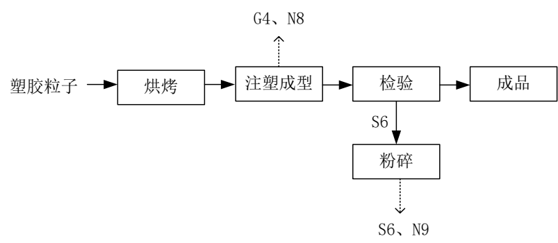
图 2-4 塑胶件生产工艺流程图
