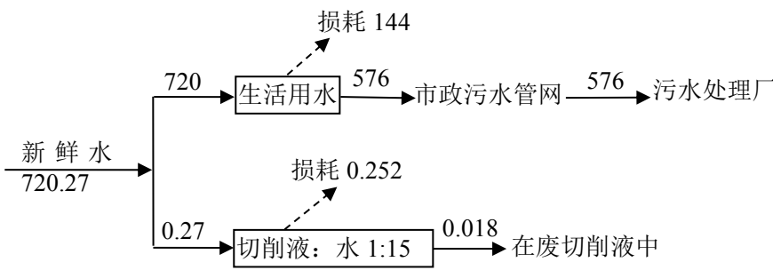
图 5-2 项目水平衡图 单位: t/a
