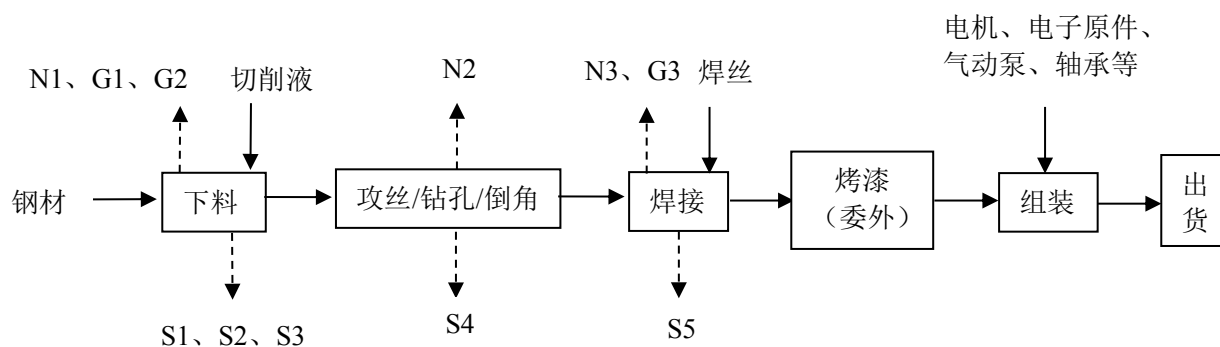
图 5-1 生产工艺流程及产污环节
