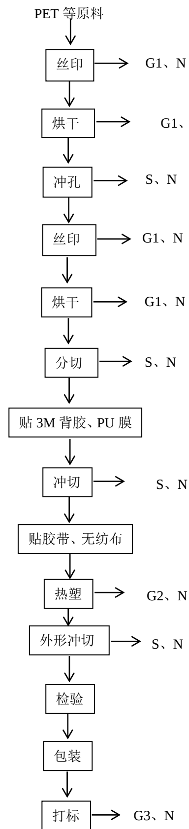
图例：G、废气； S：固废； N：噪声 图 2-1 加工工艺流程及产污环节图
