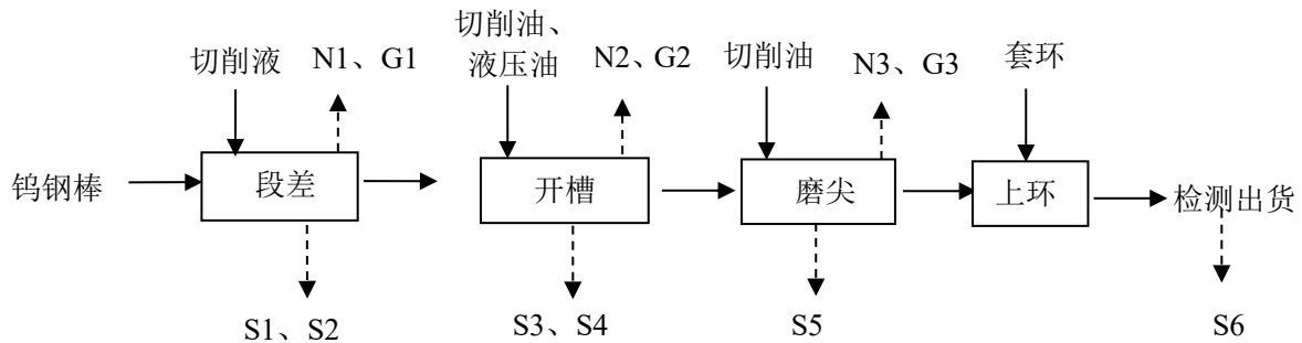
图 5-1 生产工艺流程及产污环节
