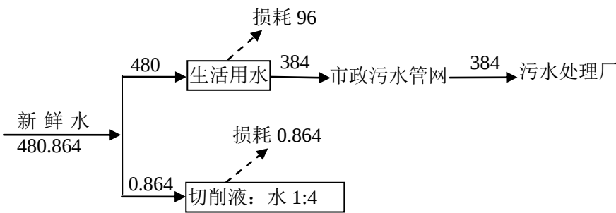
图 5-2 项目水平衡图 单位：t/a
