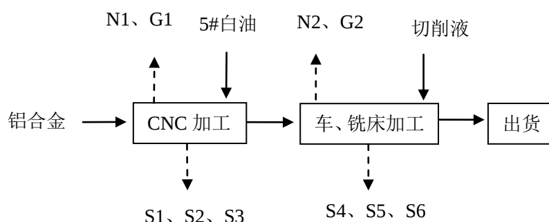
图 5-1 生产工艺流程及产污环节
