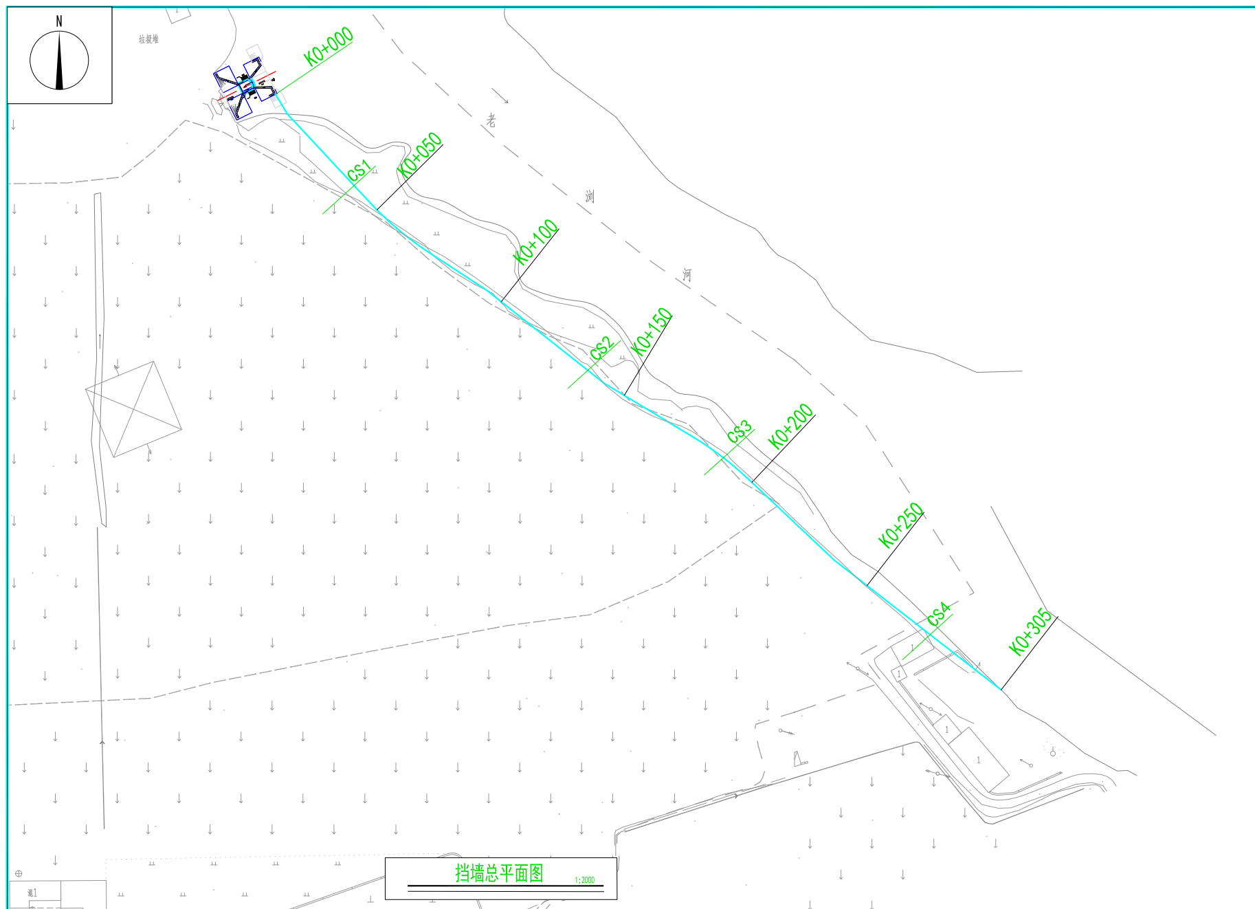
附图4-1 项目总平面图布置图（尺泾段）
