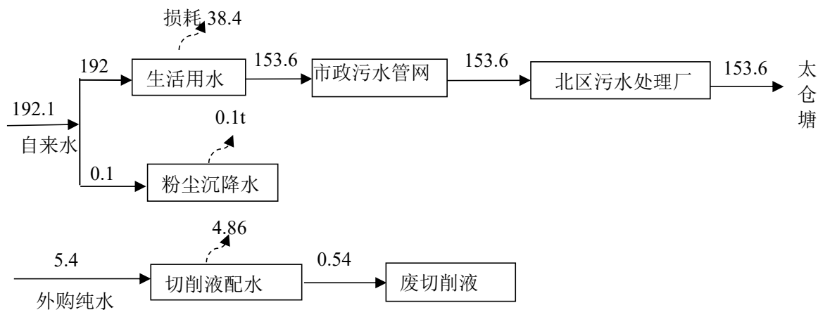
图 5-2 水平衡图 t/a
