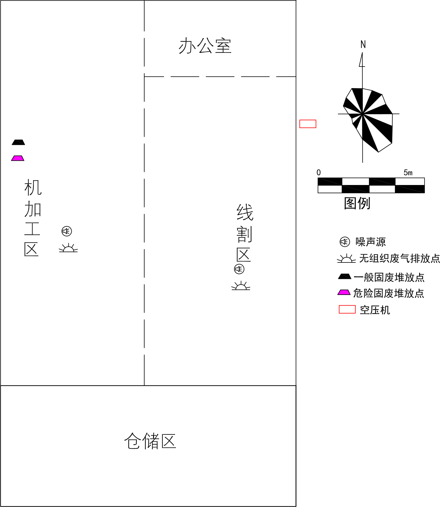
附图3 车间平面图
