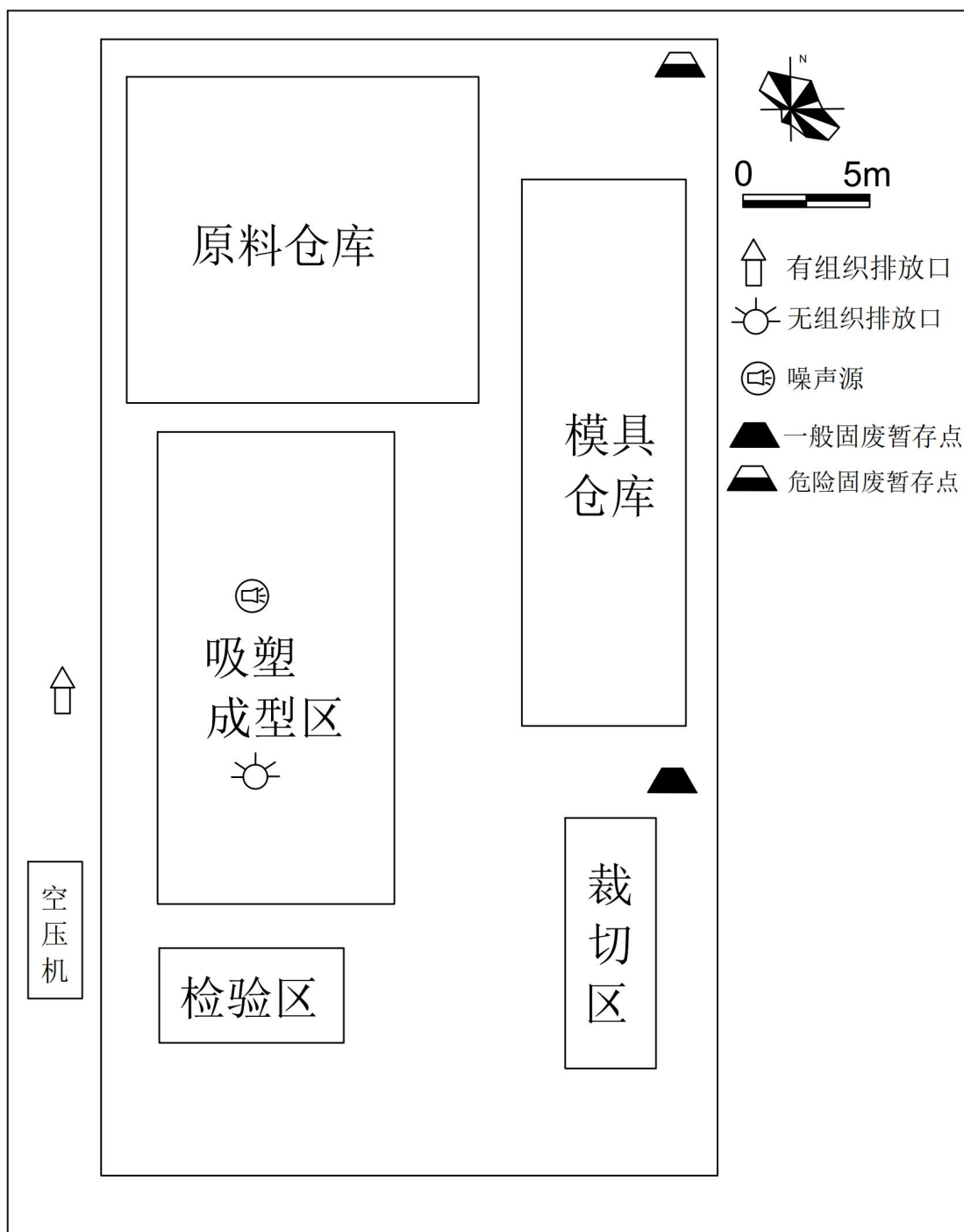
附图 3-1 项目车间一楼平面图
