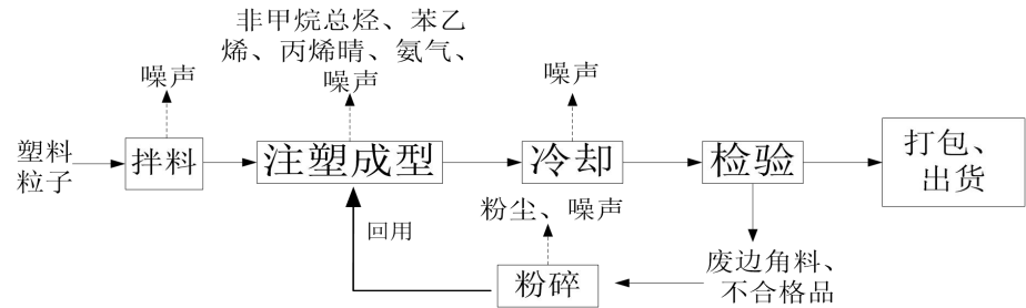
图 2-2 工艺流程图
