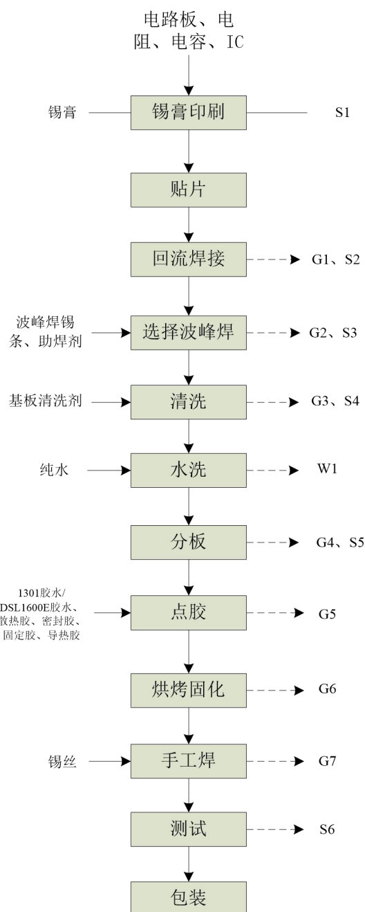
图 2-2 项目主要生产工艺流程及产污环节图
