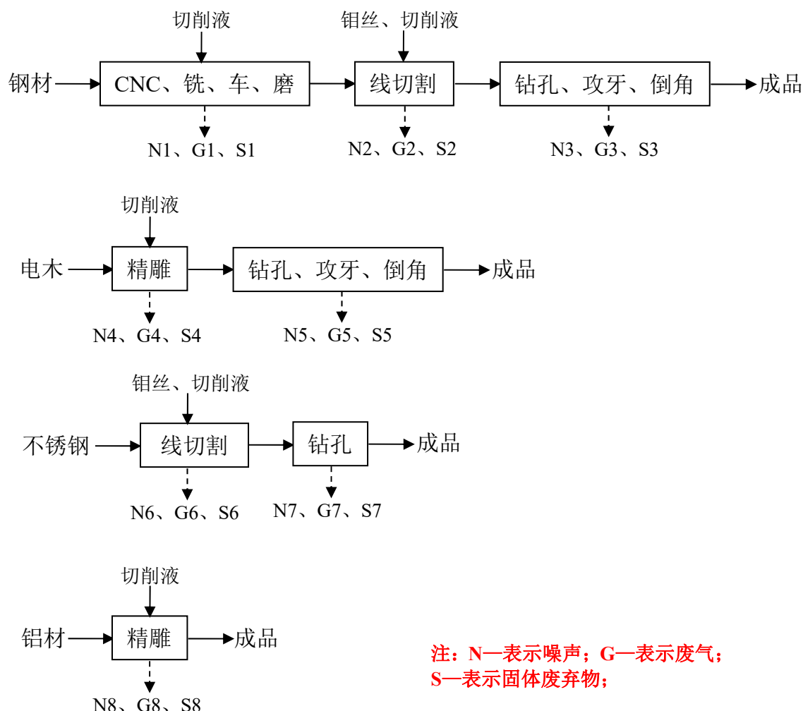
图 5-1 治具生产工艺流程及产污环节图
