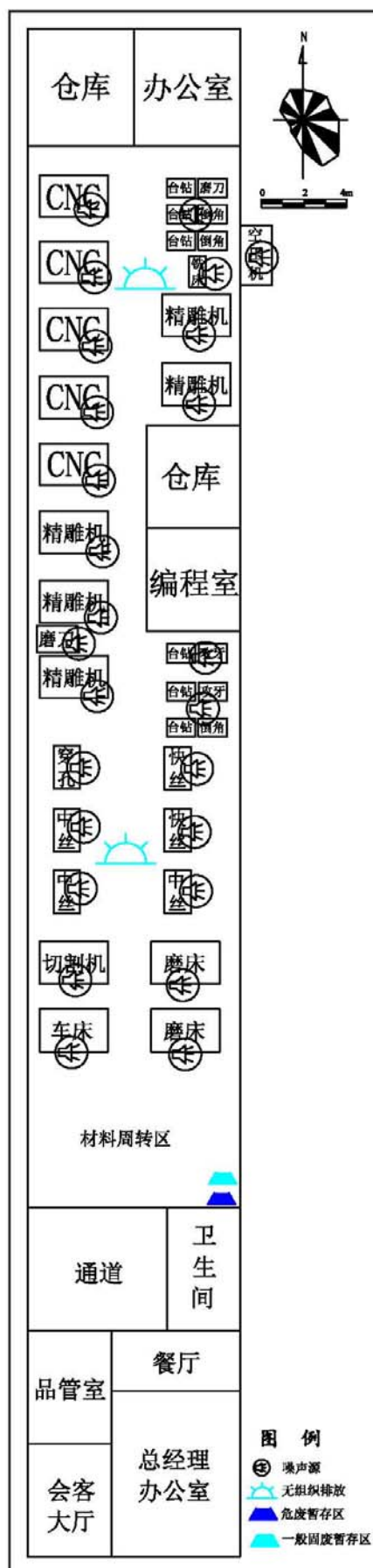
附图4 车间平面布置图
