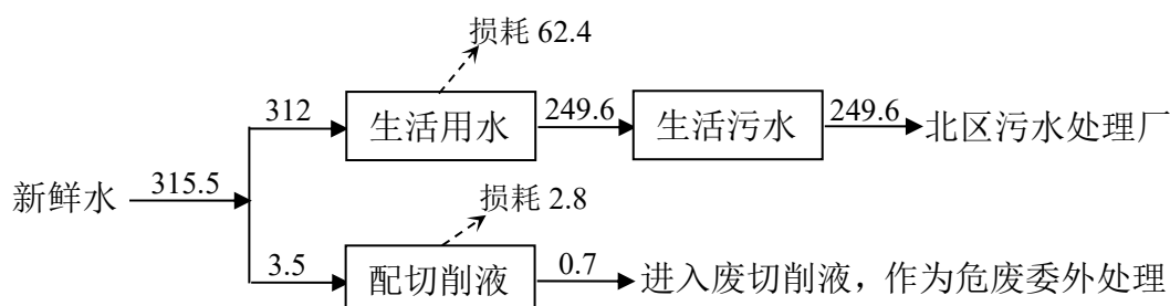
图 5-2 项目水平衡图 (单位: t/a)
