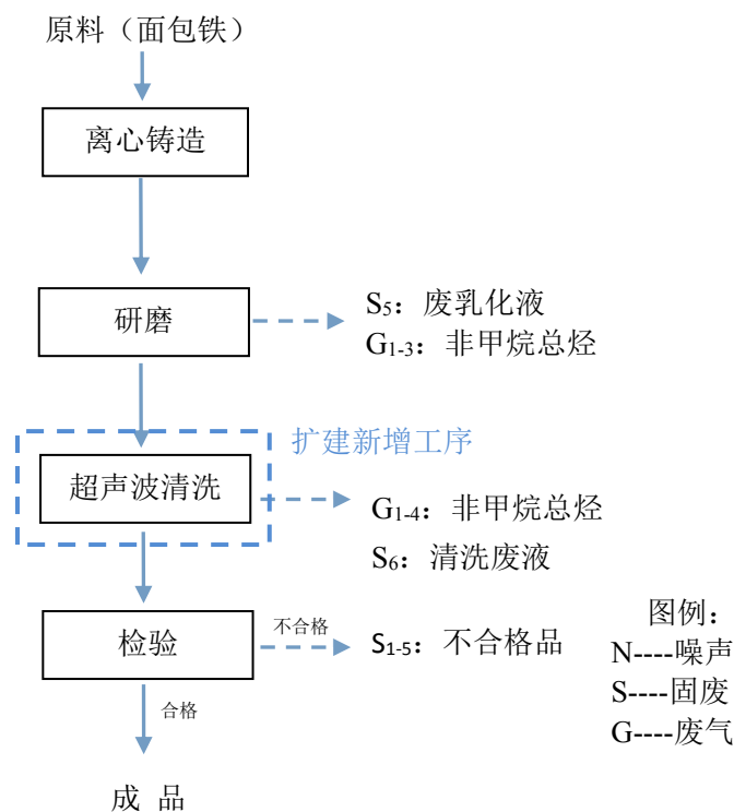
图 2-4 浮动油封工艺流程及产污环节图
