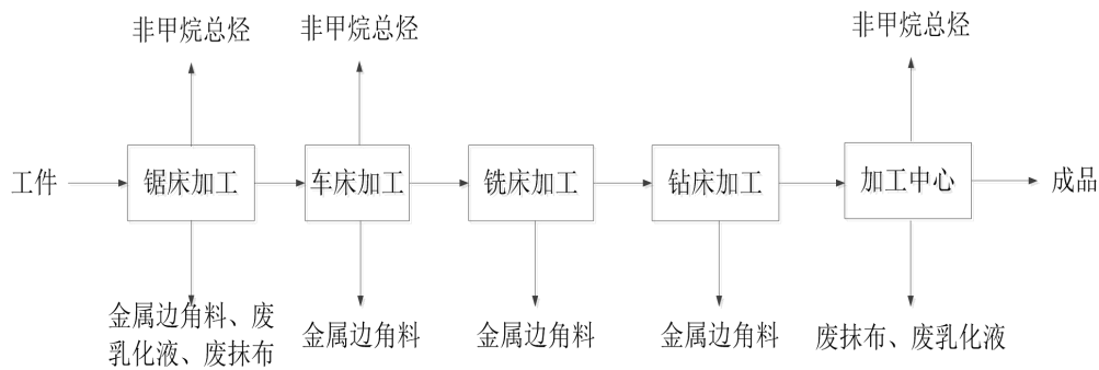
图 2-6 机加工工艺流程图及产污环节图
