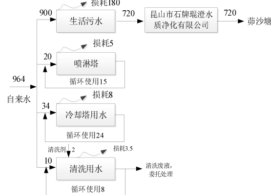
图2-1 扩建项目用排水平衡图（单位：t/a）
