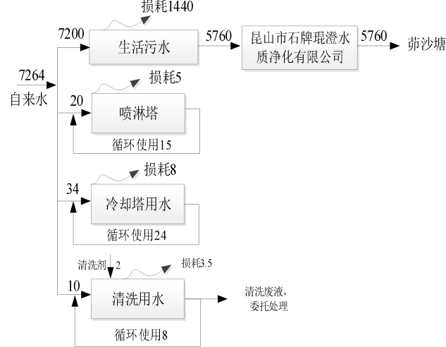
扩建项目建成后全厂用排水平衡情况见图2-2。
