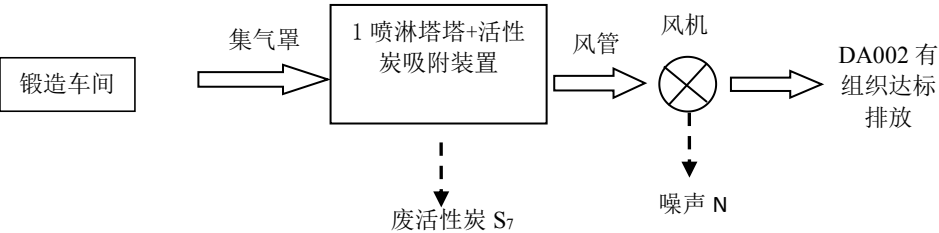
图 2-6 生产车间废气收集治理流程及产污环节图
