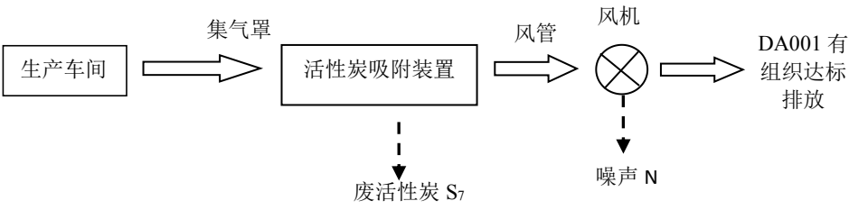
图 2-5 生产车间废气收集治理流程及产污环节图
