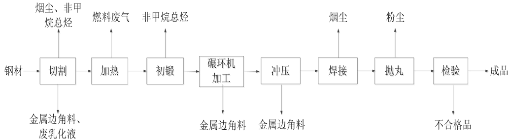
图 2-7 铁件制品工艺流程图及产污环节图
