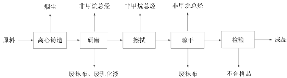
图 2-8 浮动油封工艺流程图及产污环节图
