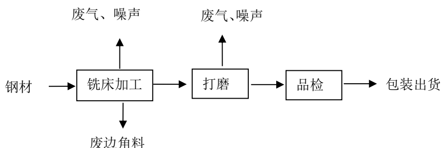
图 1-1 模具部件工艺流程及产污环节图
