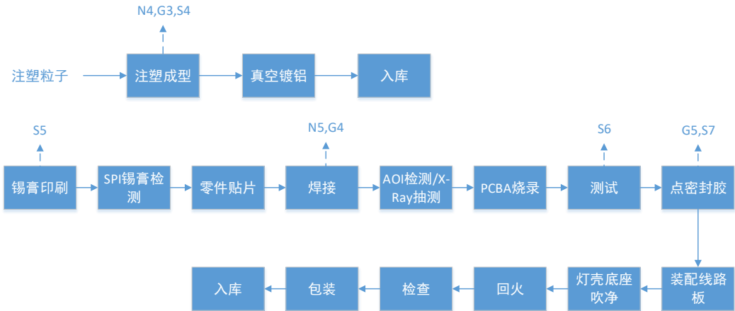
图 2-4 汽车高科技灯具生产工艺流程图
