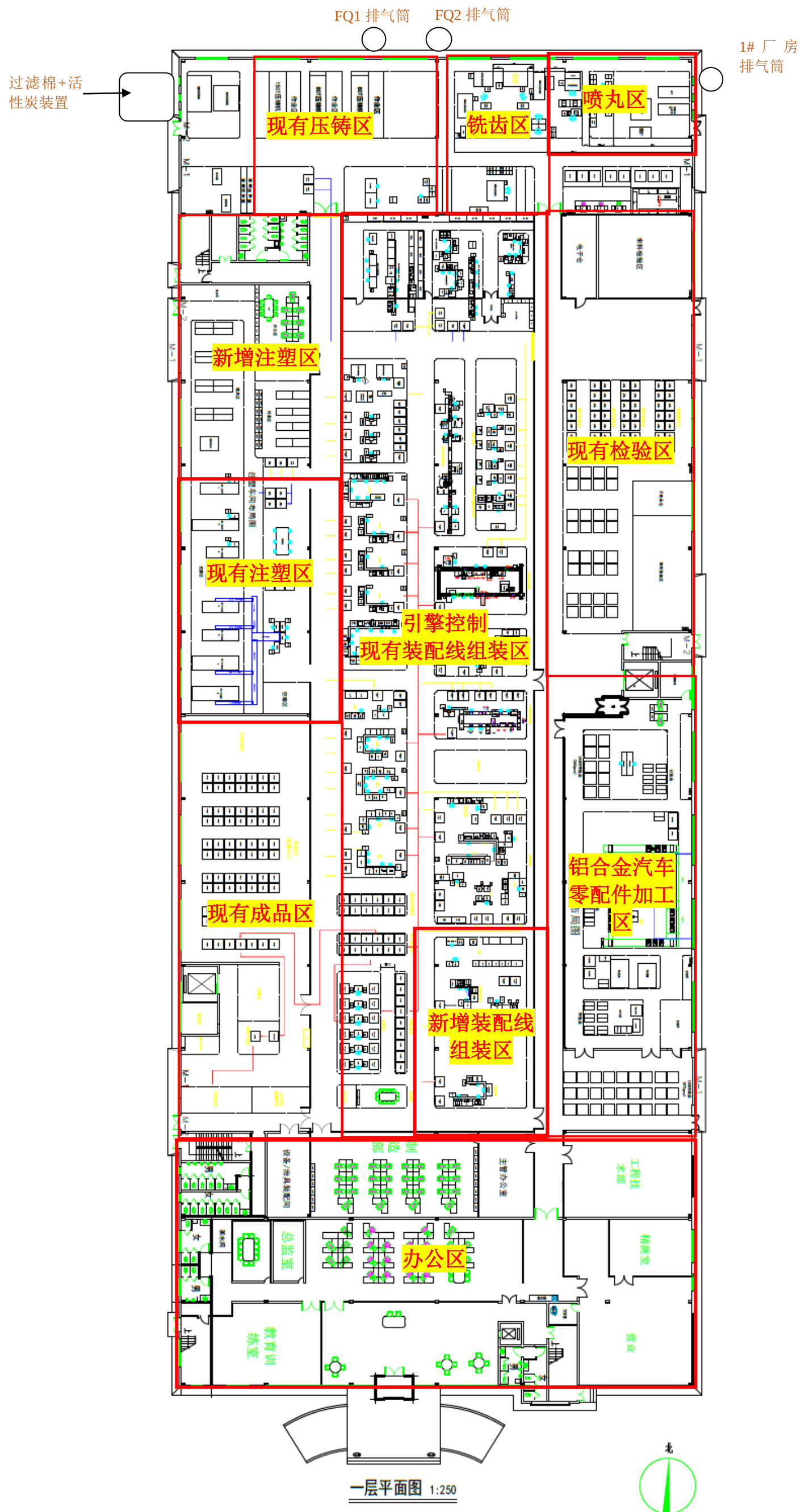
附图 8-1 1#厂房一楼车间平面布置图
