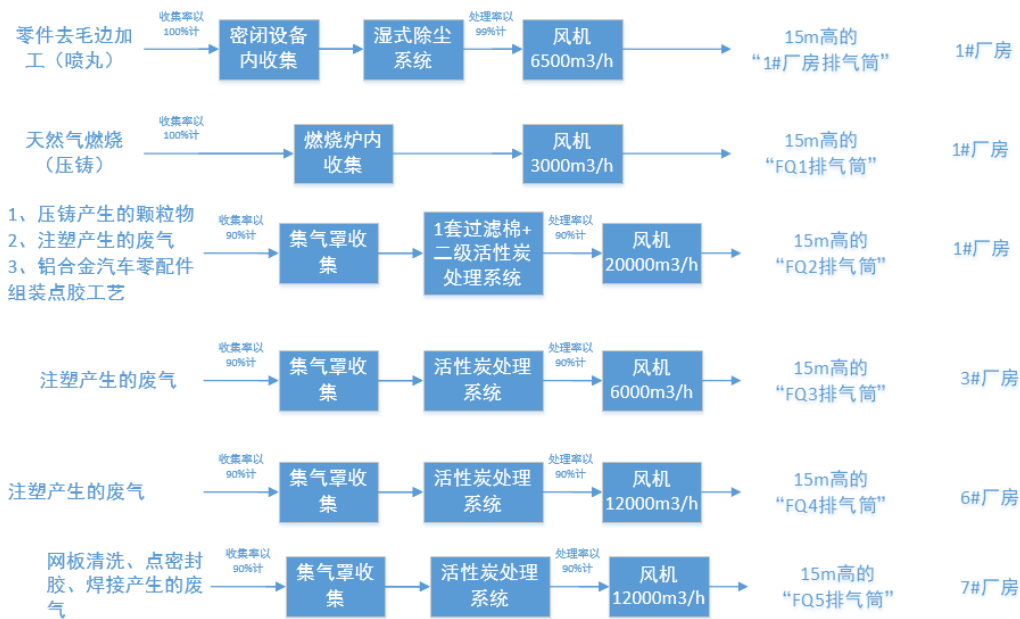
图 1.4.1 全厂废气处理流向图
