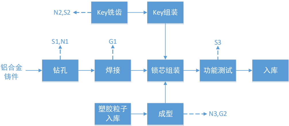
图 2-3 引擎控制生产工艺流程图
