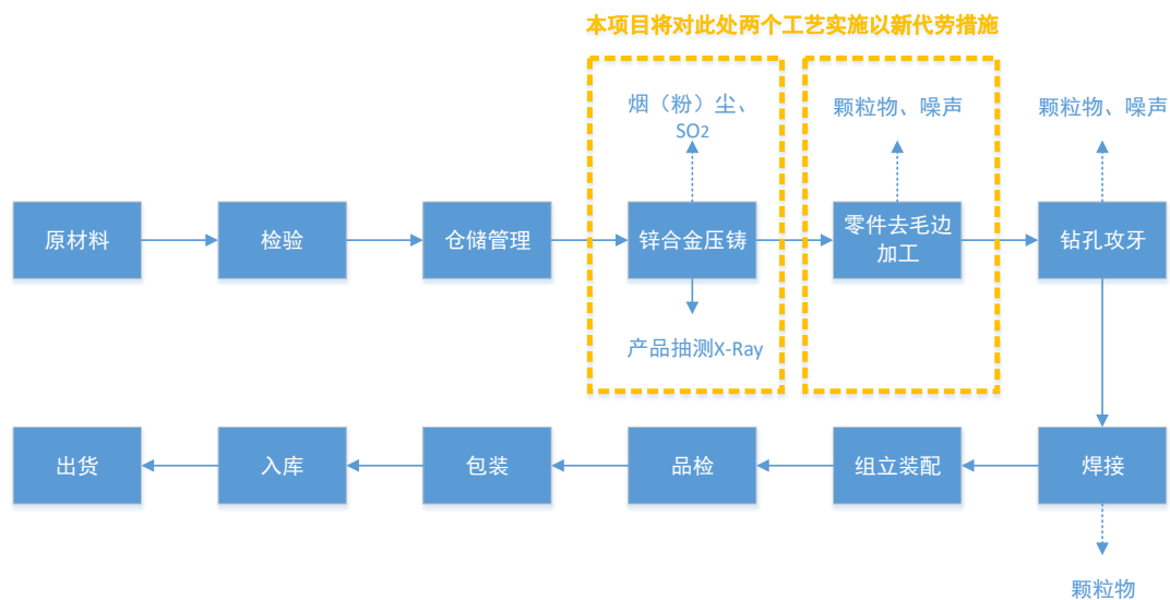
图2-6 工艺流程及产污环节
