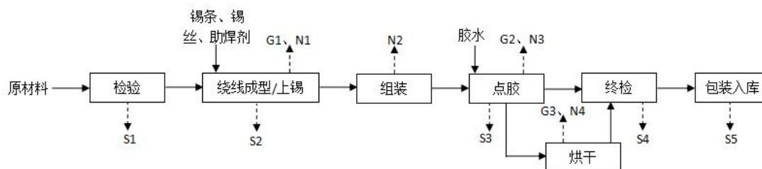
图 1-1 标准电感工艺流程及产污环节
