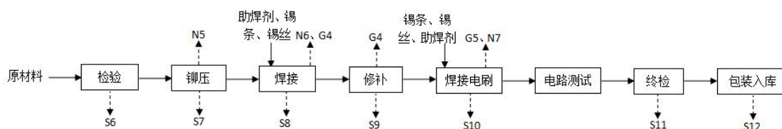
图 1-2 刷架工艺流程及产污环节
