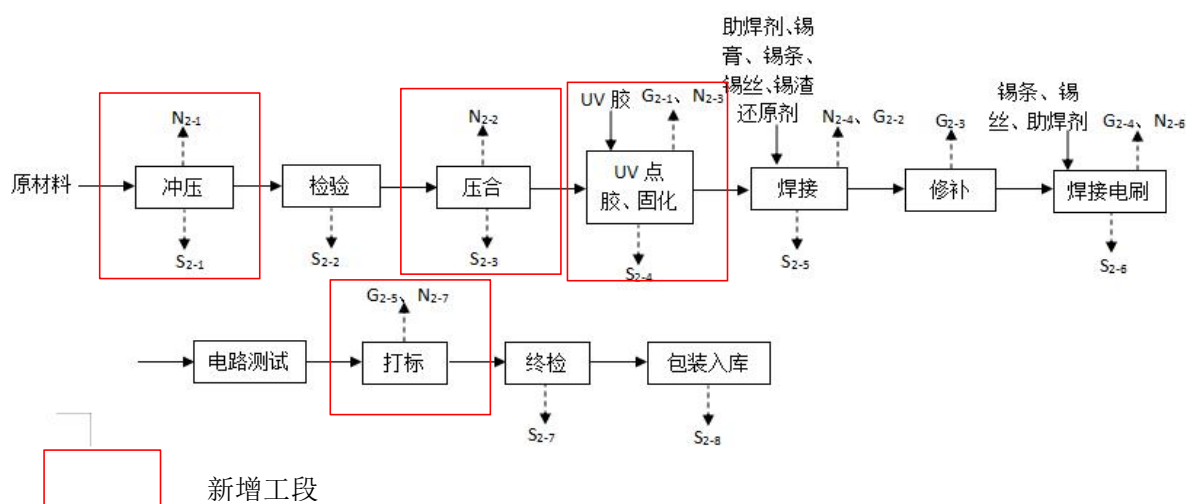
图 5-2 电机刷架生产工艺流程及产污环节图
