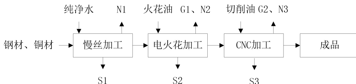
图 5-1 生产工艺流程及产污环节
