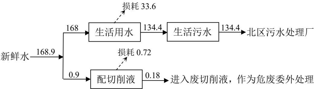
图 5-2 项目水平衡图（单位：t/a）
