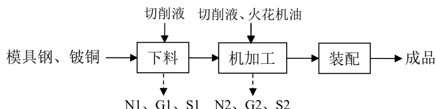
图 5-1 五金配件生产工艺流程及产污环节图
