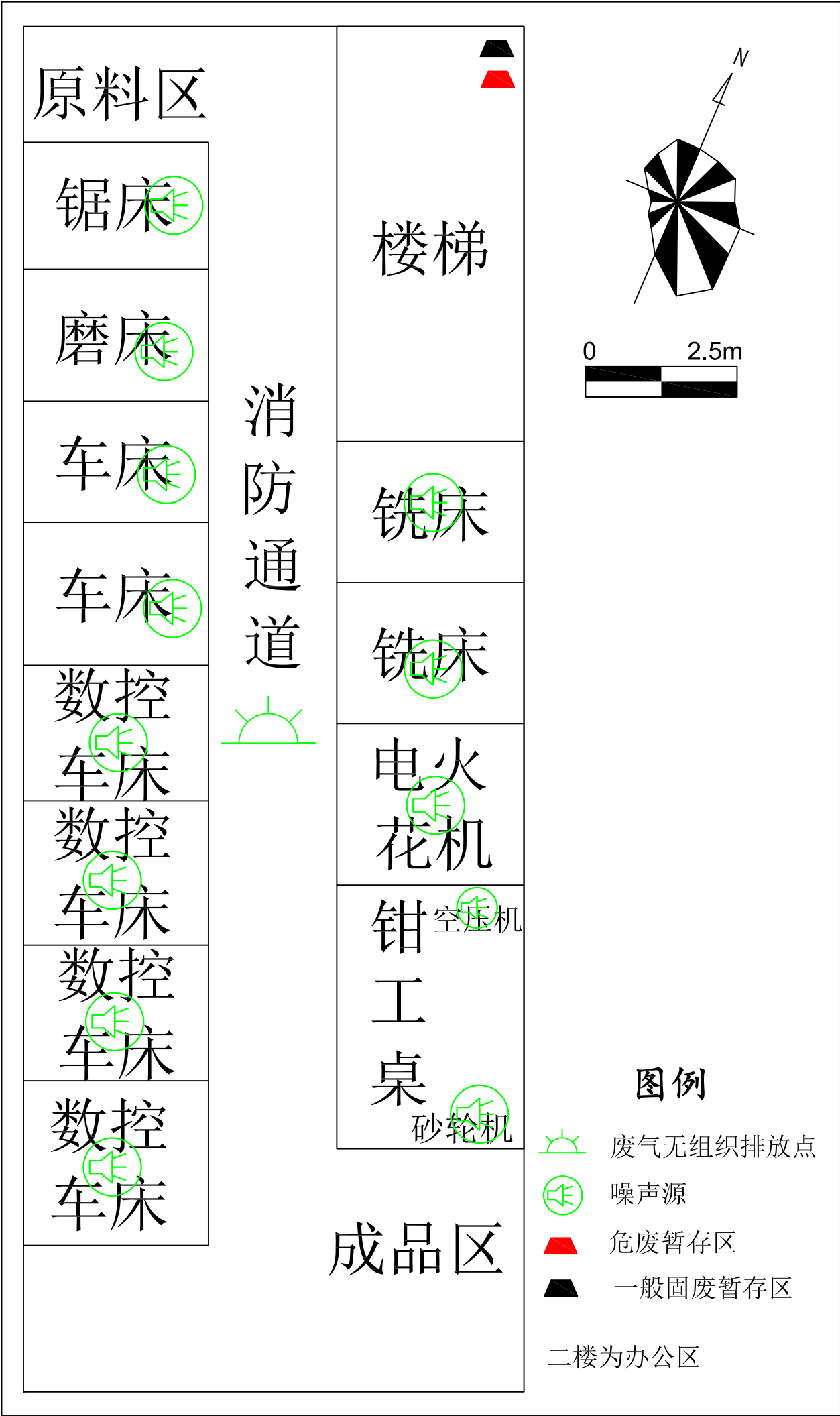
附图3 车间平面布置图
