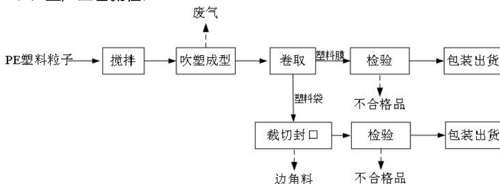
图 2-3 原项目生产工艺流程及产污环节图
