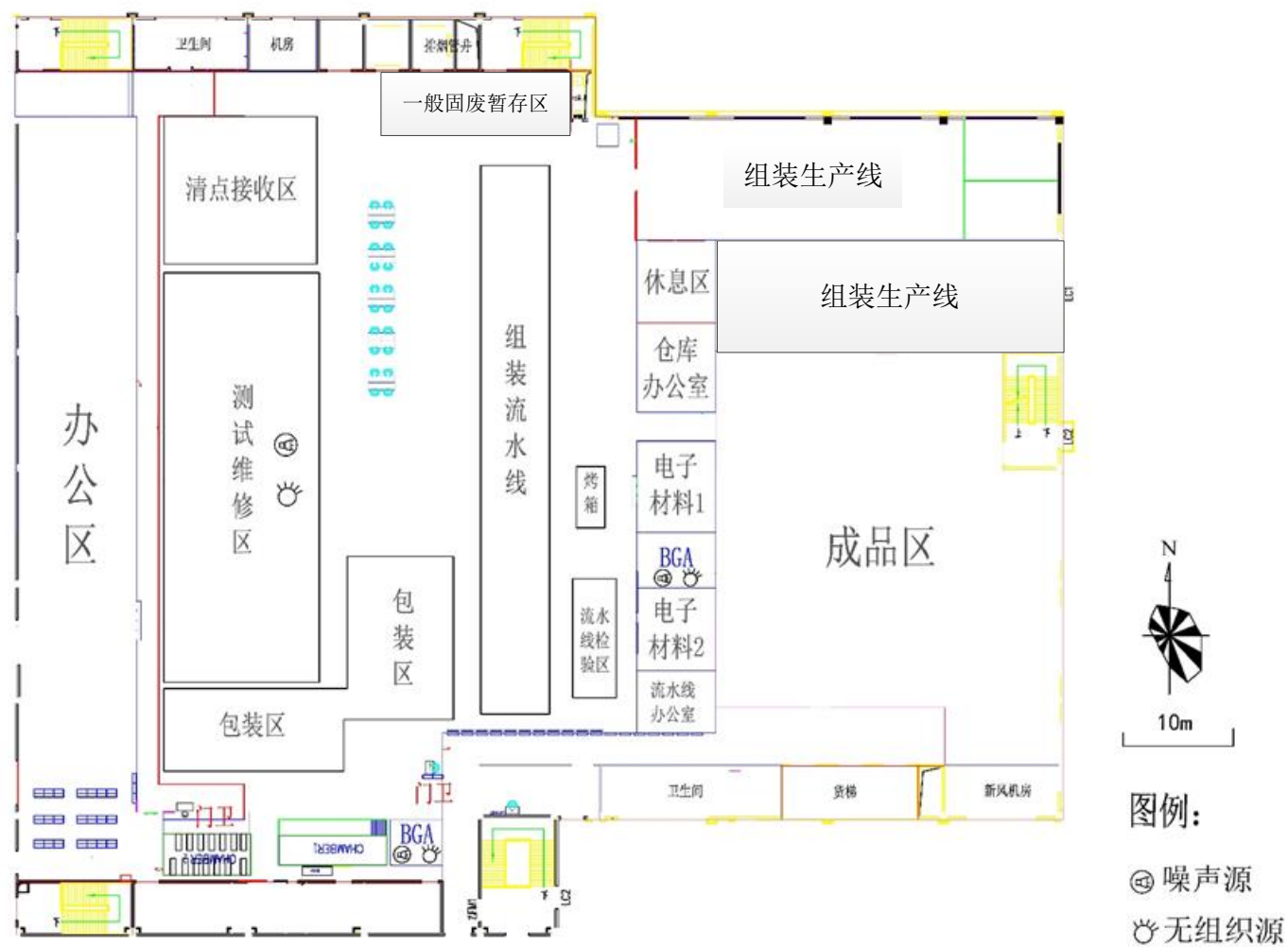
附图5 项目所在厂房平面布置图
