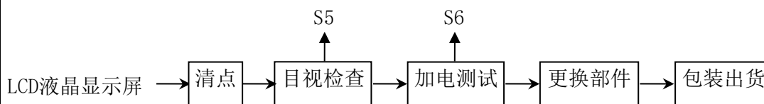
图2-3 LCD液晶显示屏加工工艺流程
