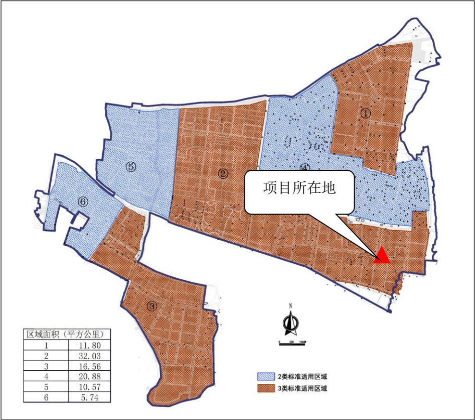
附图1 开发区声环境功能区图
