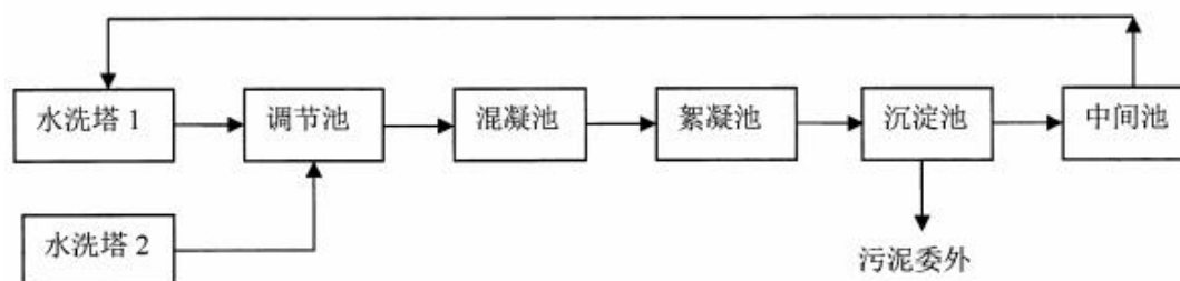
图 2-6 废水处理站 2#废水处理工艺
