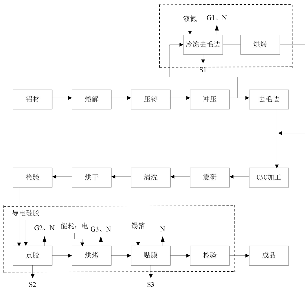
图 2-2 工艺流程图
