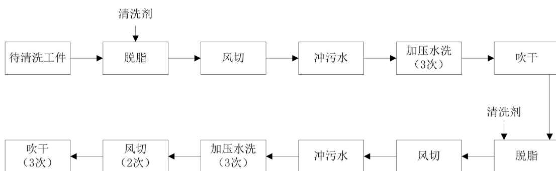
图 2-4 清洗工段工艺流程及产污环节图
