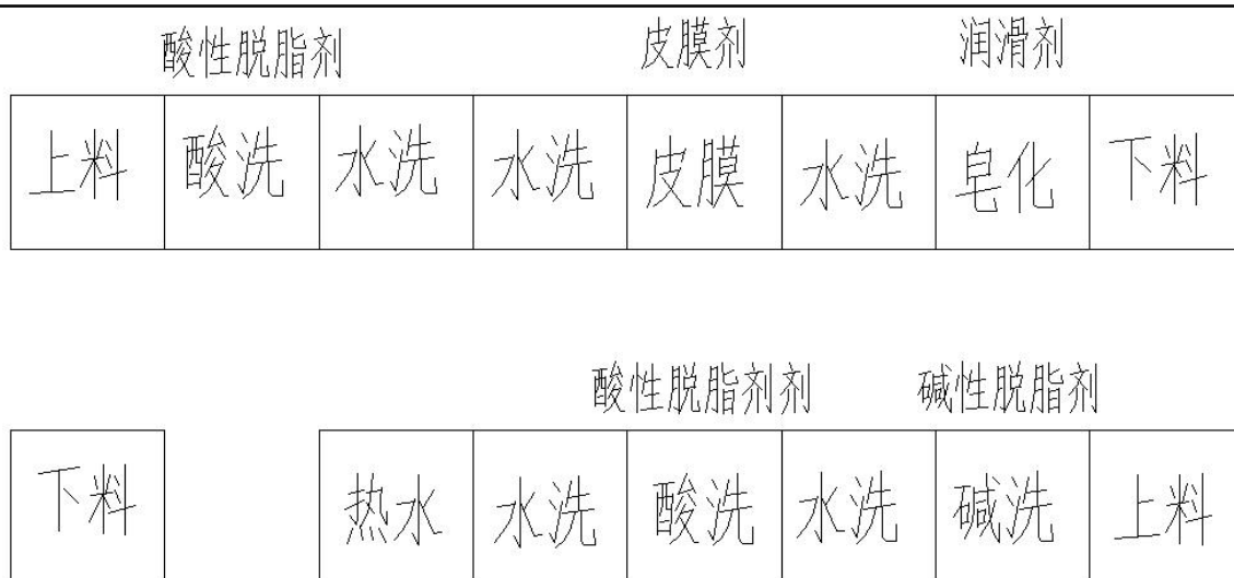
图 2-2（b） 项目清洗工艺流程图
