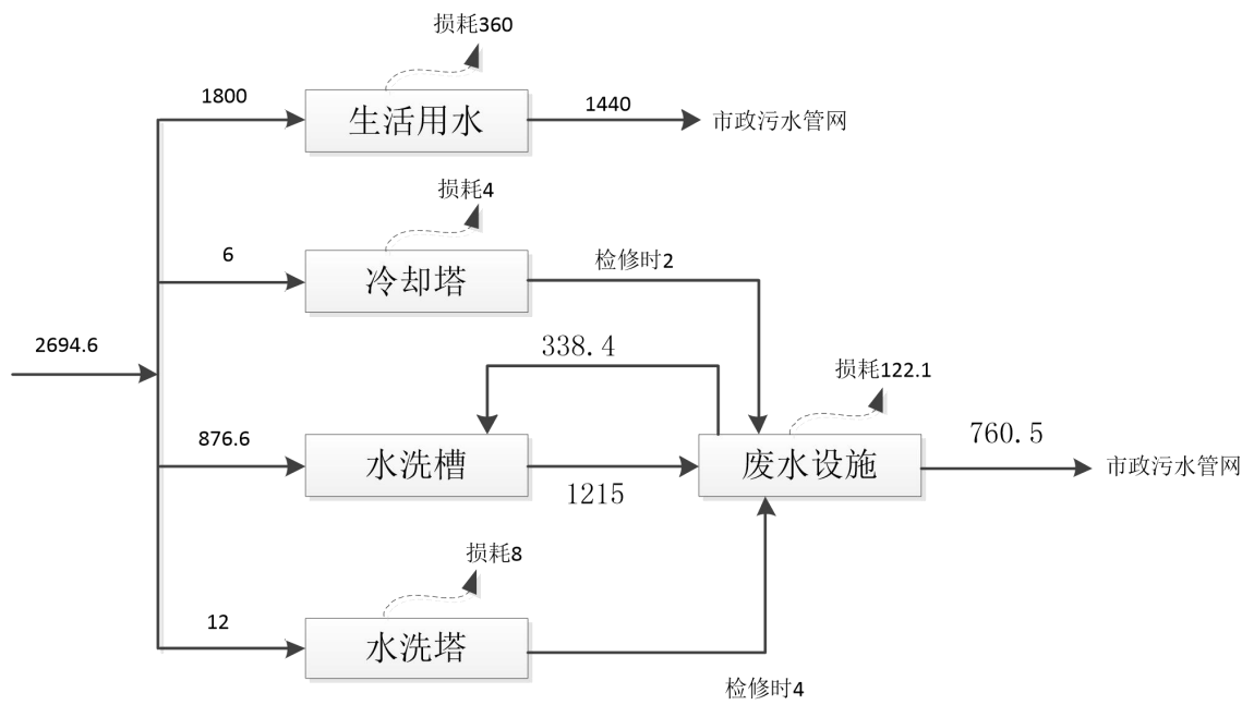
图 2-1 项目迁建后水量平衡图
