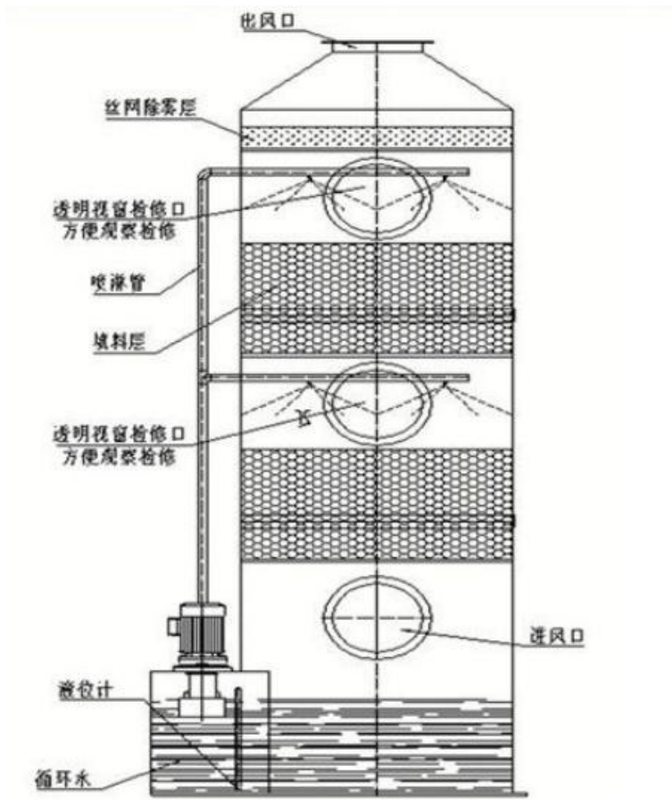
图 4-1 喷淋塔结构示意图
