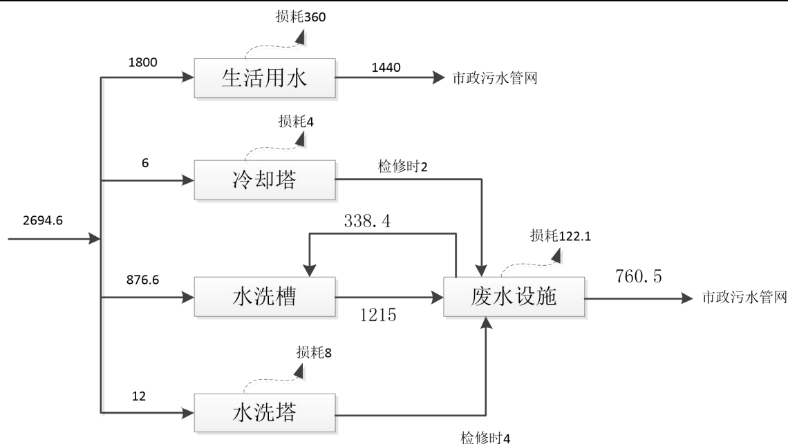
图 4-2 (b) 项目迁建后水量平衡图
