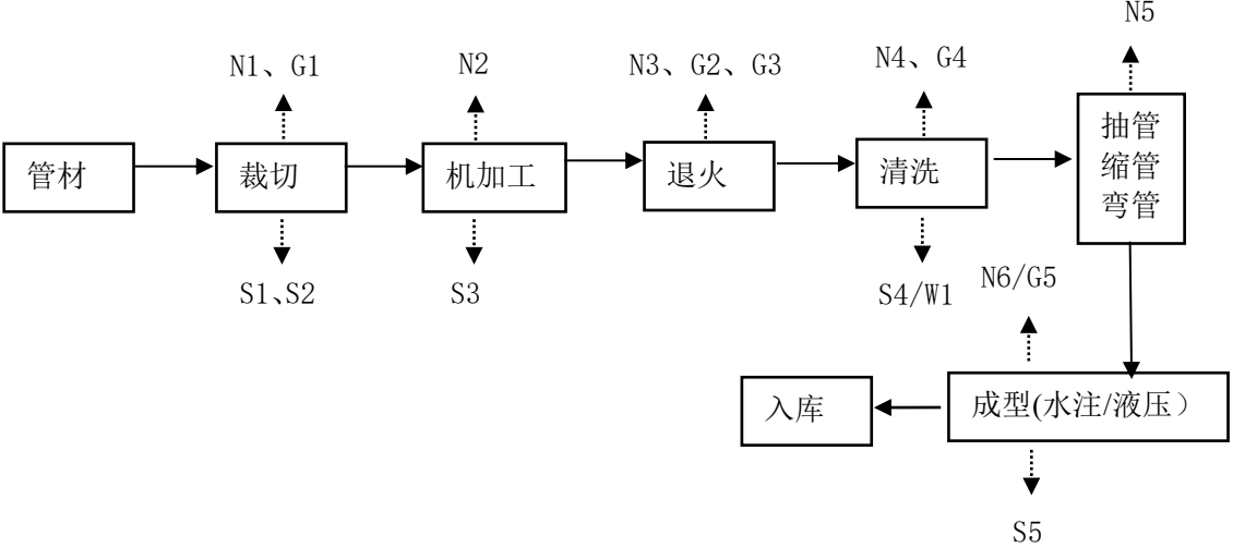
图 2-2（a） 项目生产工艺流程图
