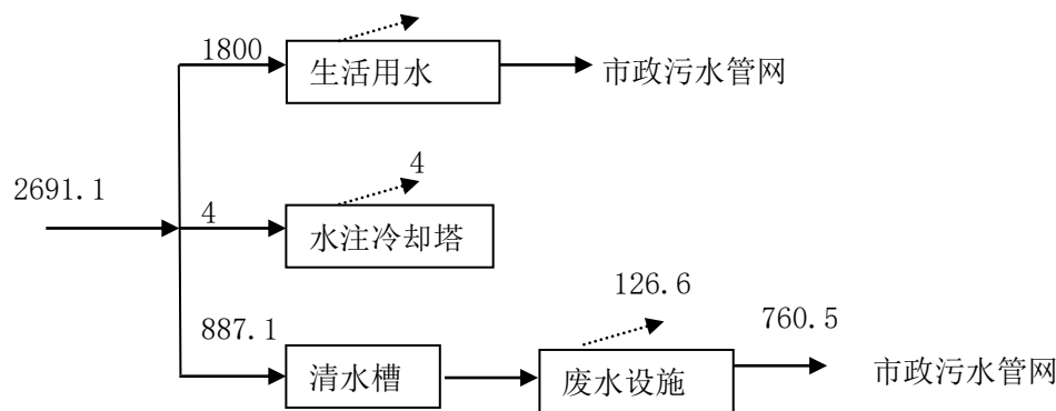
图 4-2（a） 项目迁建前水量平衡图
