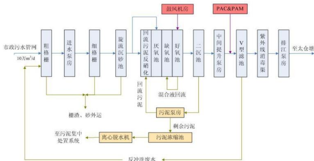
图 4-4 北区污水处理厂现有一、二期工艺流程图
