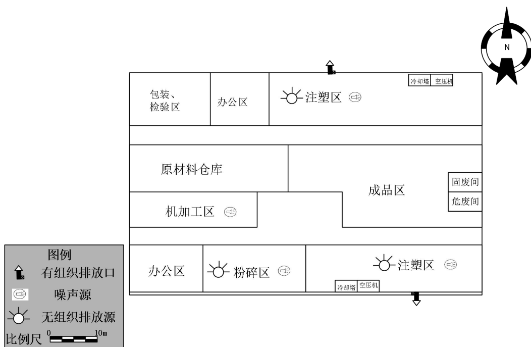
附图 3 车间平面布置图
