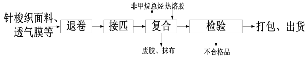
图 2-2 复合面料工艺流程及产污环节图
