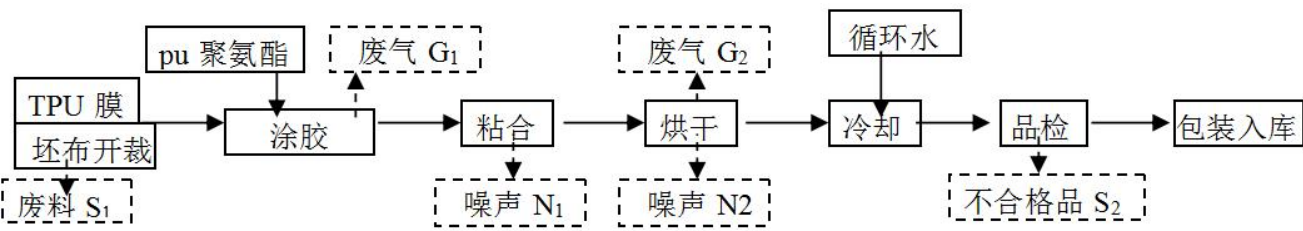
图 2-3 原项目高档透气布料生产工艺流程及产污环节图
