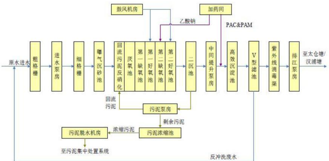
图 4-2 昆山建邦环境投资有限公司北区污水厂三期、四期工艺流程
