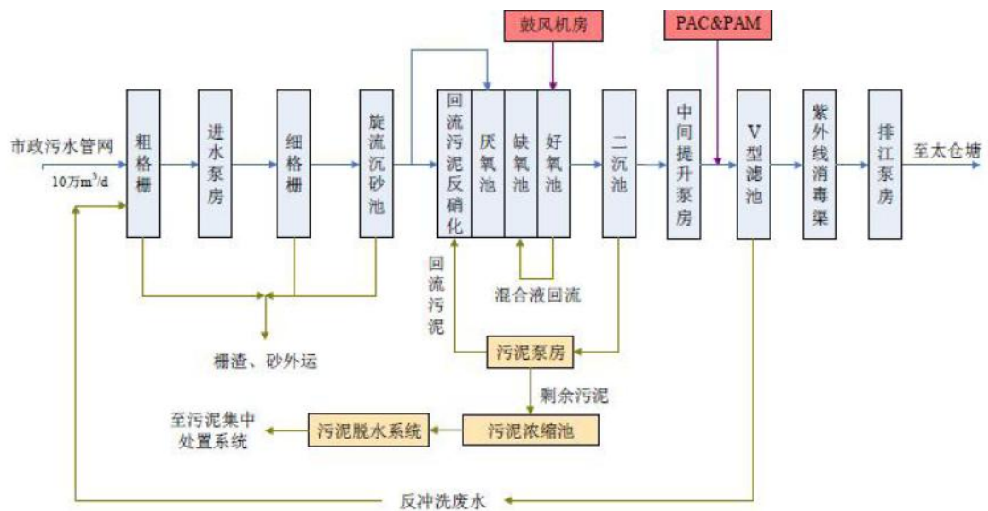
图 4-1 昆山建邦环境投资有限公司北区污水厂一期、二期工艺流程
