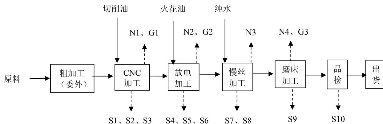
图 5-1 生产工艺流程及产污环节
