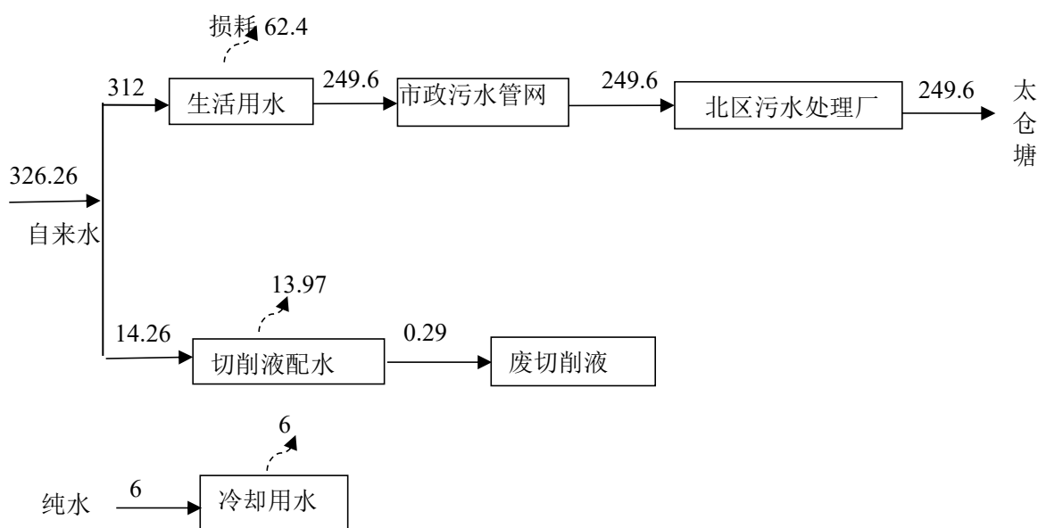
图 5-2 水平衡图 t/a
