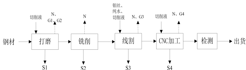
图 5-1 生产工艺流程及产污环节
