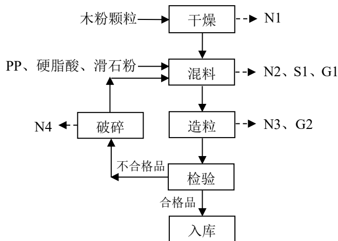
图 2-4 木塑颗粒生产工艺产污环节流程图
