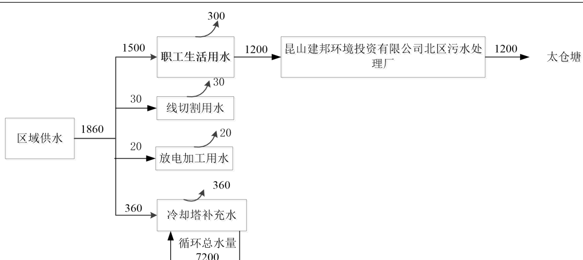
图 2-1 项目新建后全厂水平衡图(t/a)
