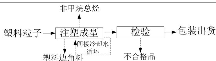
图 5-2 本项目塑胶配件生产工艺流程及产污环节图
